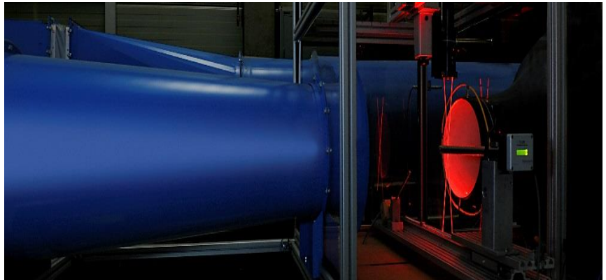
Freistrahl-Windkanal WK320 mit Laser-Doppler-Anemometer (LDA)
